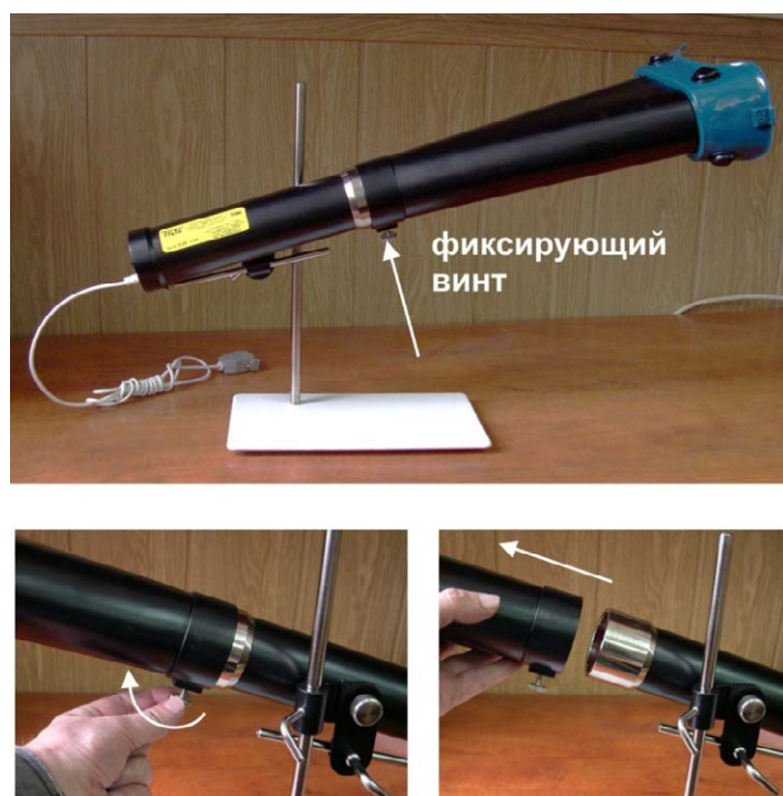
Рис.6. Снятие дополнительного тубуса с приставки.
